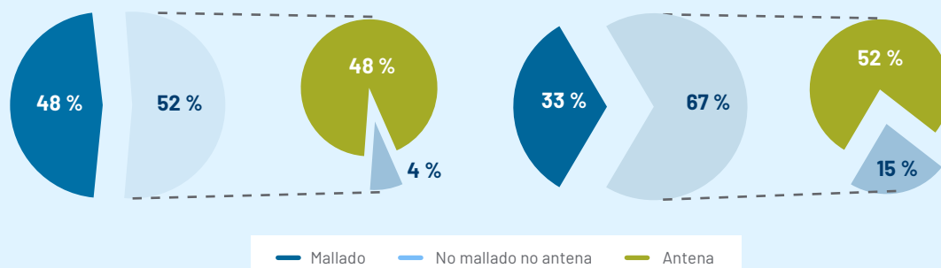
Figura 27. Topología y número de interrupciones por topología en los sistemas eléctricos balear y canarios
