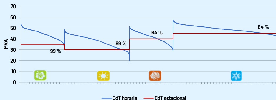
Figura 18. Representación gráfica de la máxima capacidad de transporte obtenida con DLR
