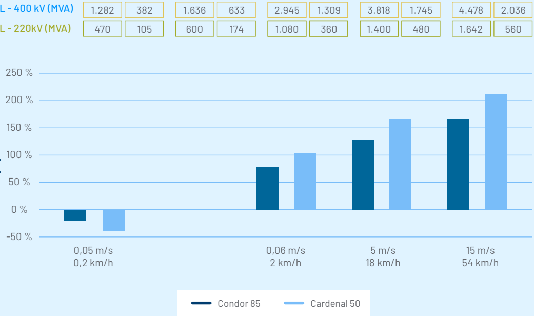
Figura 20. Influencia del viento en la capacidad de transporte de las líneas
