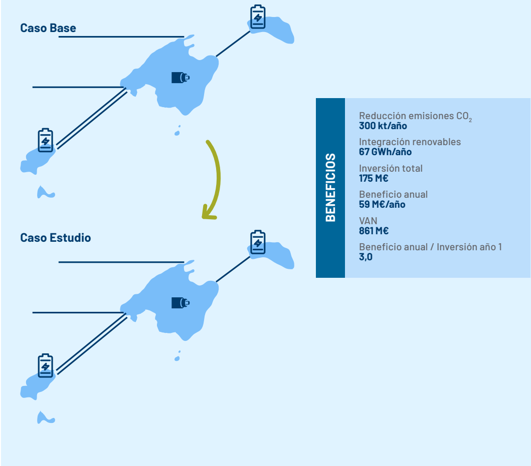
Figura 34. Análisis CBA de los CS con segundo HVDC y con baterías
