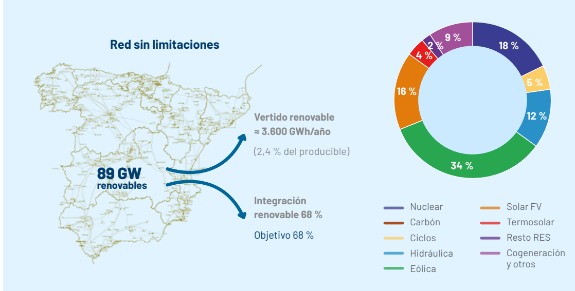
Figura 33. Principales resultados de un escenario que cuente sólo con una red sin limitaciones. El gráfico circular representa la contribución de cada tecnología a la cobertura de la demanda
