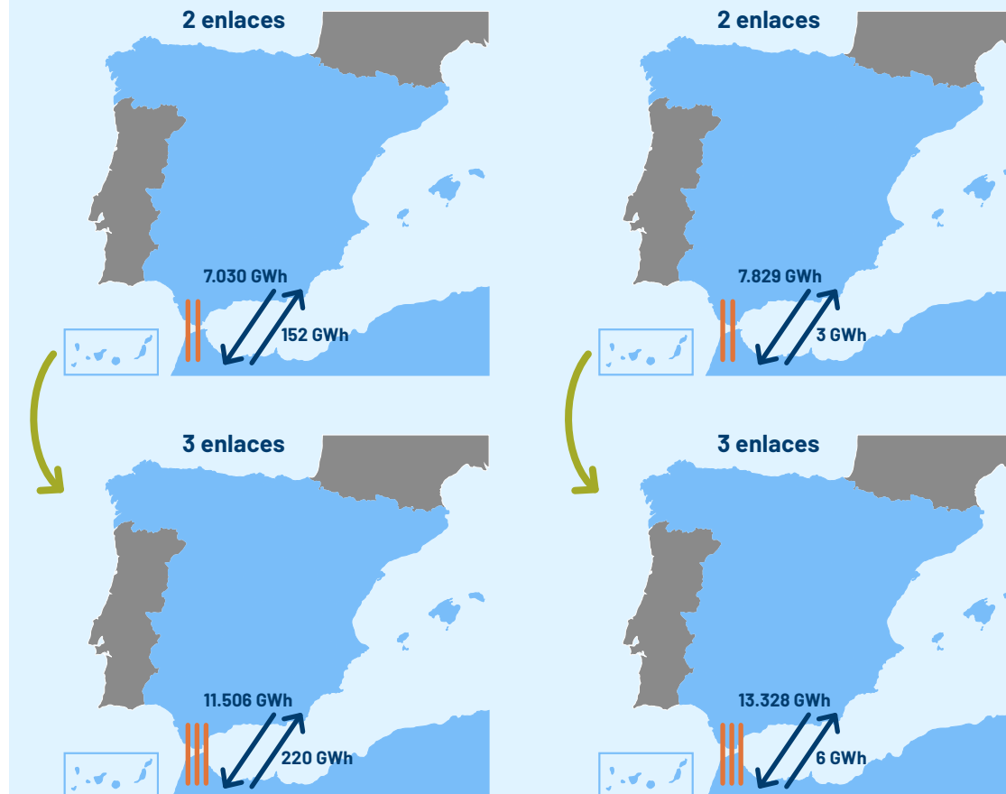
Figura 38. Impacto en intercambios de un tercer enlace con Marruecos en 2026 (izda.) y 2030 (dcha.)
