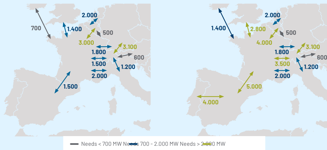
Figura 27. Necesidades de incremento de capacidad más allá de Golfo de Vizcaya e interconexión norte a 2030 (izda.) y 2040 (dcha.)
