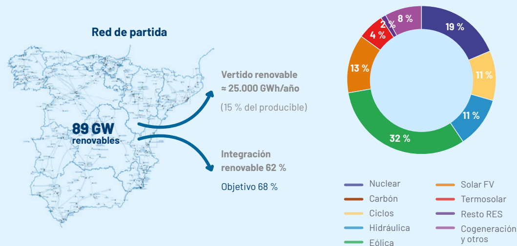
Figura 32. Principales resultados de un escenario que cuente sólo con la red de partida. El gráfico circular representa la contribución de cada tecnología a la cobertura de la demanda
